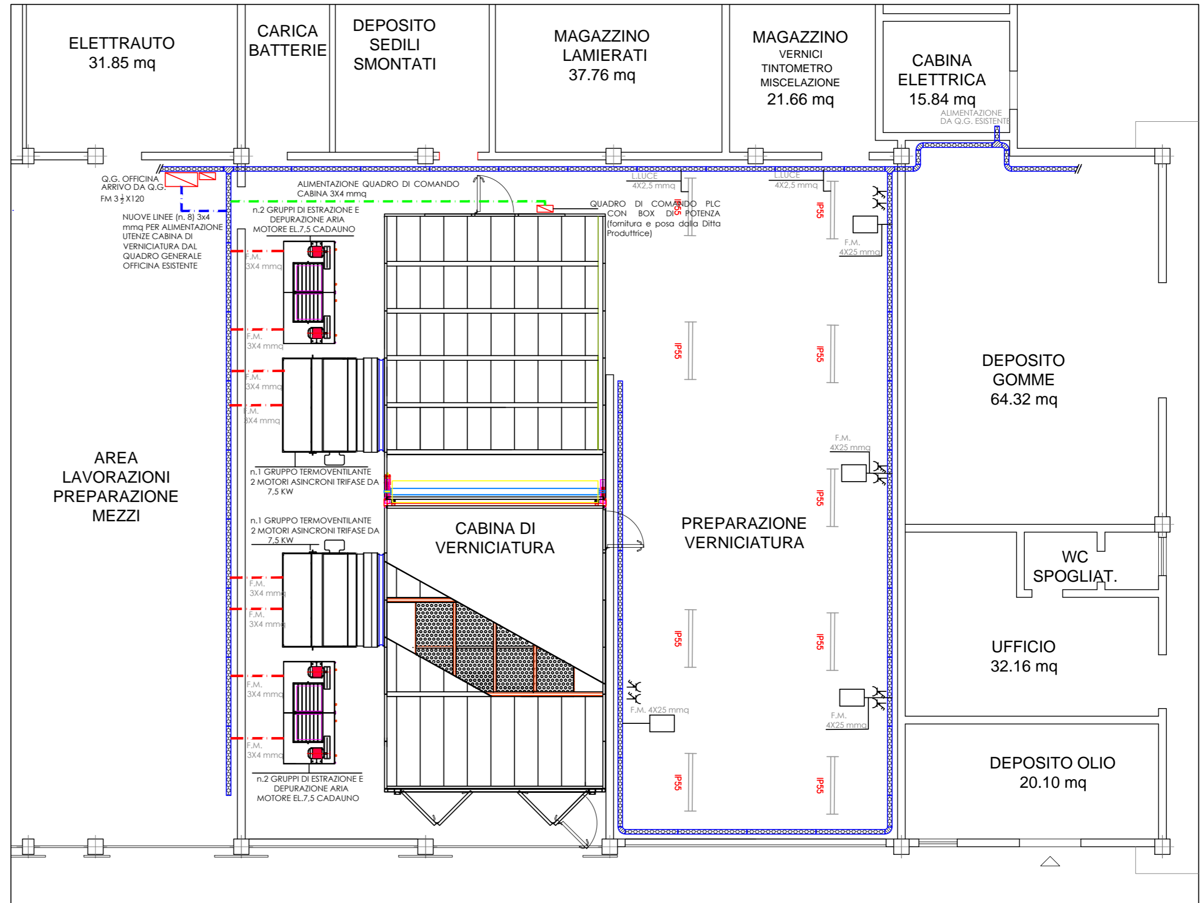
ZONA OGGETTO DI INTERVENTO_NUOVE LINEE DI ALIMENTAZIONE ELETTRICHE
